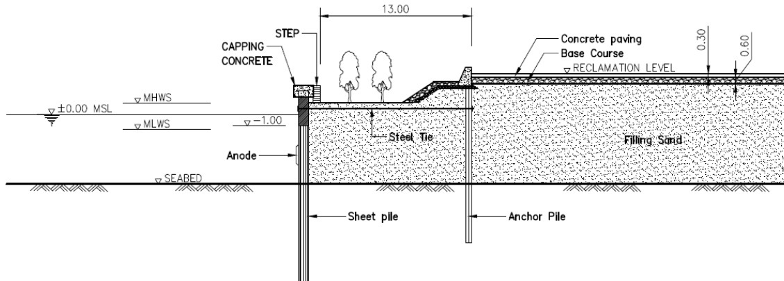
รูปที่ 7 ภาพตัดโครงสร้างเสาเข็มเหล็กพืด (Steel Sheet Pile Wall)
